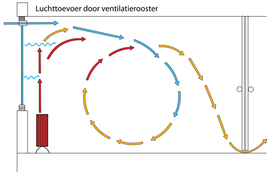
Koudeval met radiator
