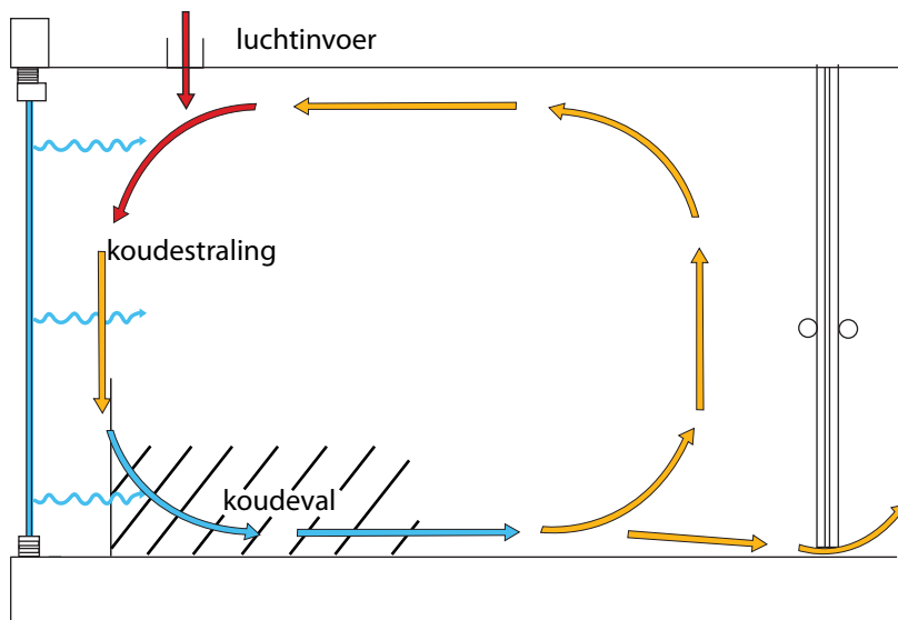
Koudeval met luchtinvoer
